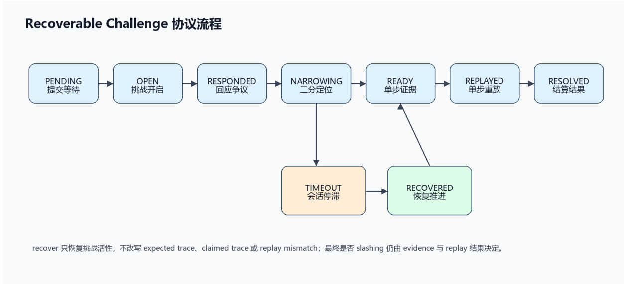
图 2 可恢复挑战协议流程
