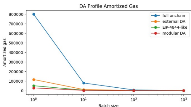
图 4 不同数据可用性配置下的摊销 gas 用量趋势 Fig.4 Amortized gas trends under different DA configurations
